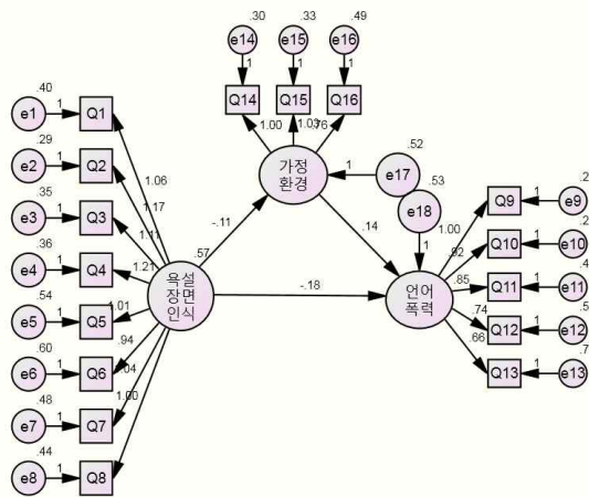
그림 3. 구조방정식모형
